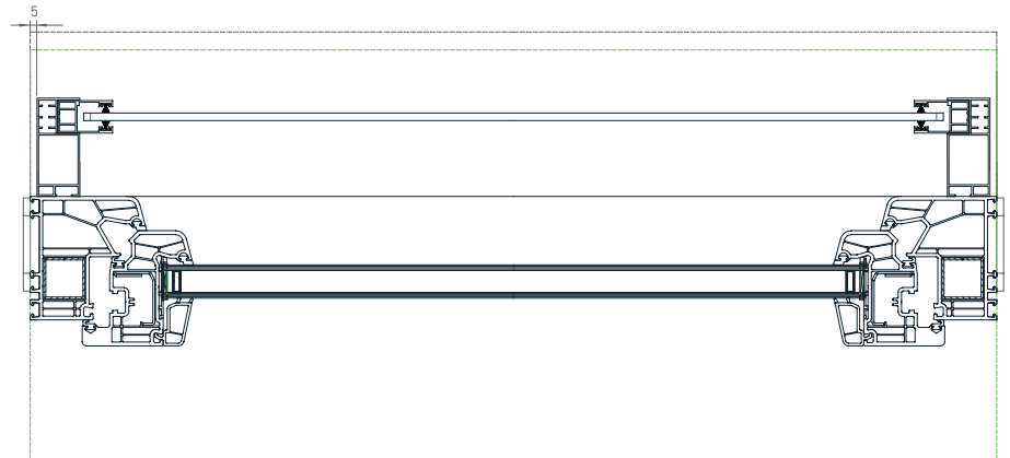
VERSETZT FÜHRUNGSSCHIENEN
