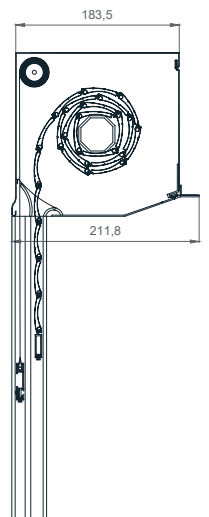
UNTERPUTZ 20° 180
