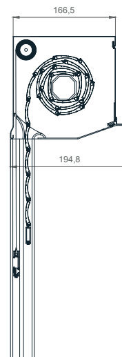
UNTERPUTZ 20° 165
