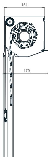
UNTERPUTZ 20° 150
