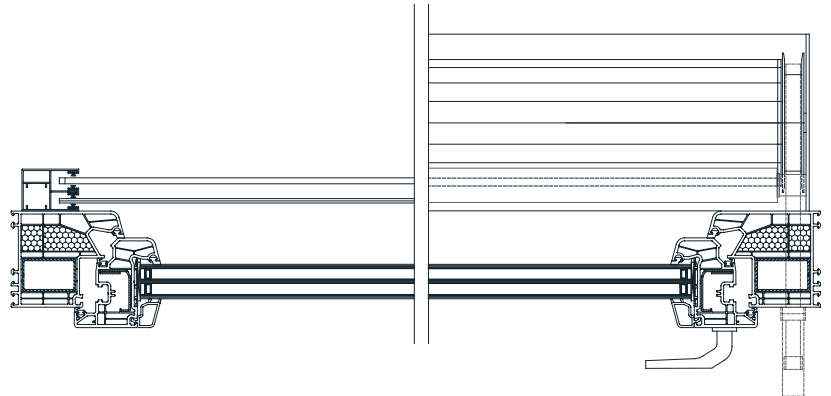
UNTERPUTZ 20° 137
