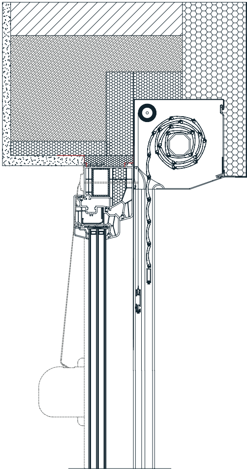
UNTERPUTZ 20° 137
