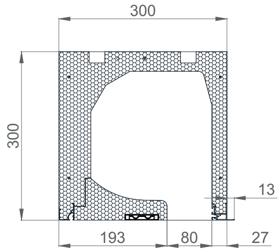
DIM. 300 X 300
